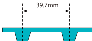
ピッチは参考サイズになります
